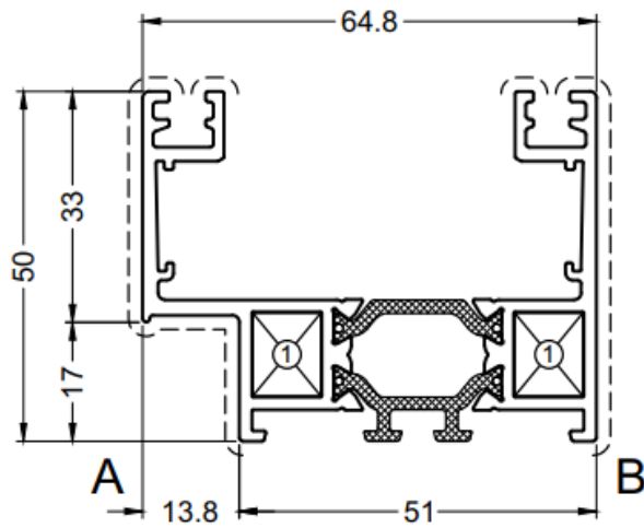
Ramprofil, 2 spår
