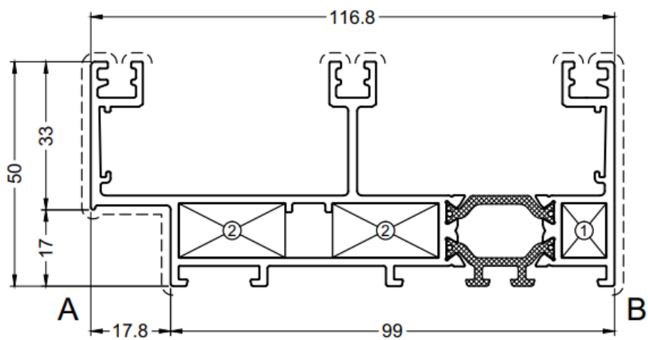
Ramprofil, 3 spår
