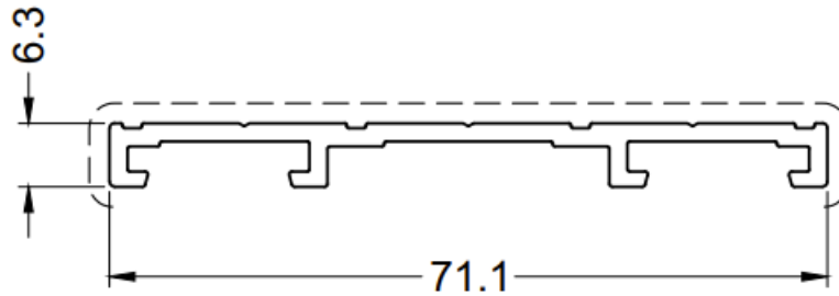
Sidoprofil, 2-delat och 3-delat (3 spår)
