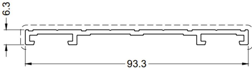
Sidoprofil, 4-delat (4 spår)
