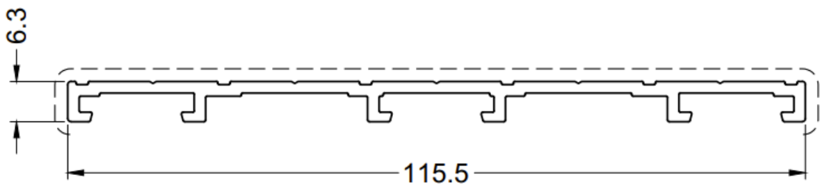
Sidoprofil, 5-delat (5 spår)
