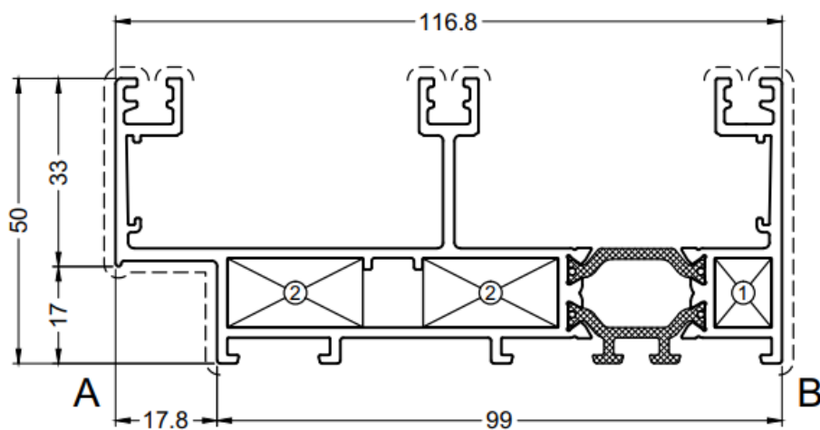
Ramprofil, 3 spår
