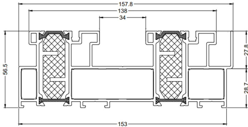
Ramprofil med 2 spår för 2 skjutbara luckor
